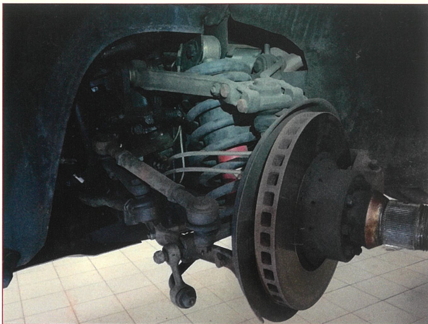
Sospensione anteriore
